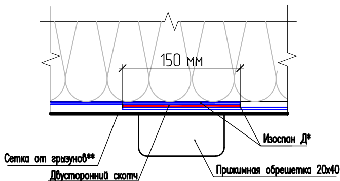
Узел № 1.
